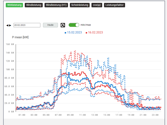
Profilo di carico con larghezza di banda di fluttuazione
