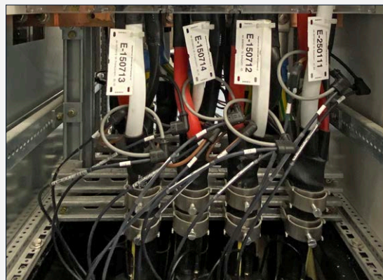
Moduli Current Link installati sul campo
