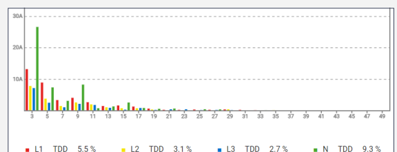
Analisi delle armoniche/interarmoniche per tutte e 4 le correnti di ciascun modulo di corrente, disponibile anche come medie a 10 minuti
