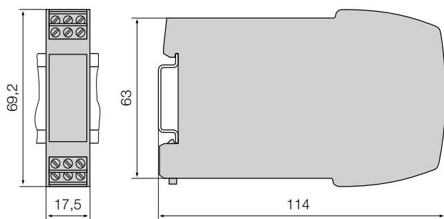
Fig. 8. SINEAX TV 819 en boîtier P12/17 encliqueté sur rail «en chapeau» (35 × 15 mm ou 35 × 7,5 mm, selon EN 50 022), bornes de raccordement pas enfichables.
