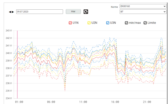
Courbes des valeurs de tension à 10 minutes
