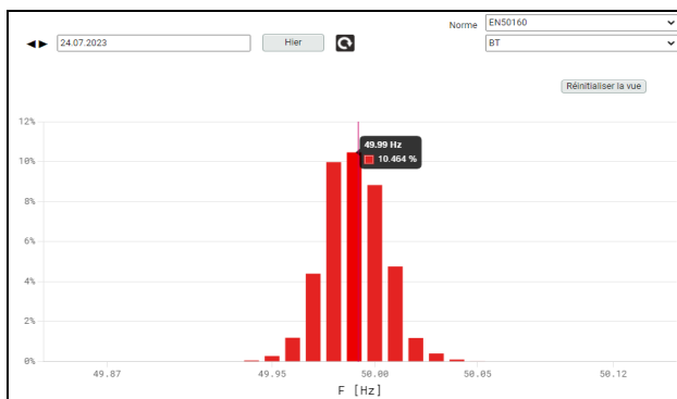
Distribution statistique des valeurs de fréquence 10-s
