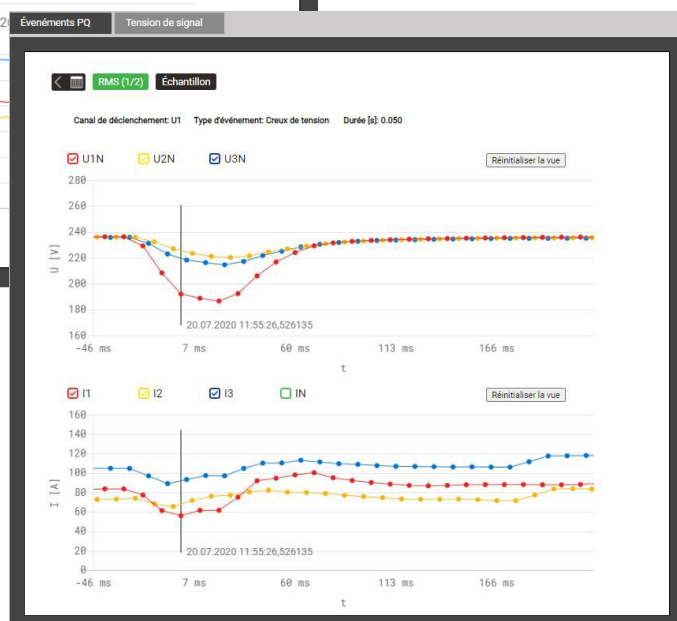
Événement PQ agrandi
