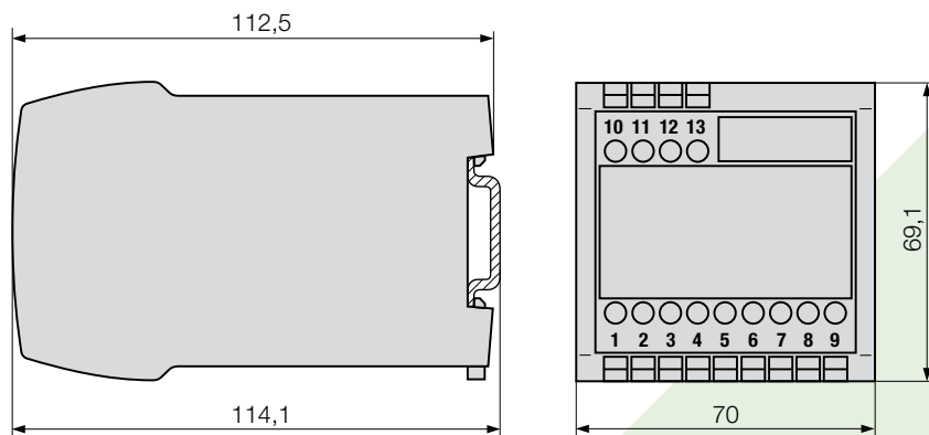
Fig. 7. SINEAX I552 en boîtier P13/70 encliqueté sur rail «à chapeau» (35 × 15 mm ou 35 × 7,5 mm, selon EN 50 022).
