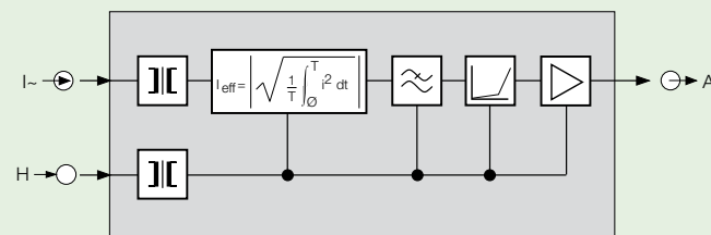
Fig. 2. Schéma fonctionnel.
