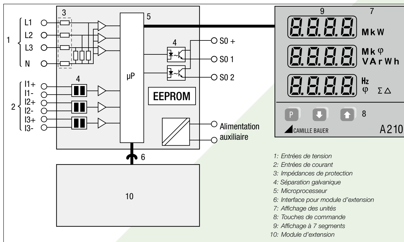
Fig. 1. Schéma fonctionnel
