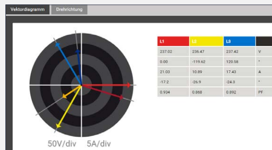
Diagramme vectoriel pour le contrôle de la connexion
