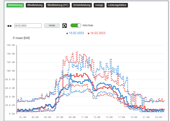
Profil de charge avec marge de fluctuation
