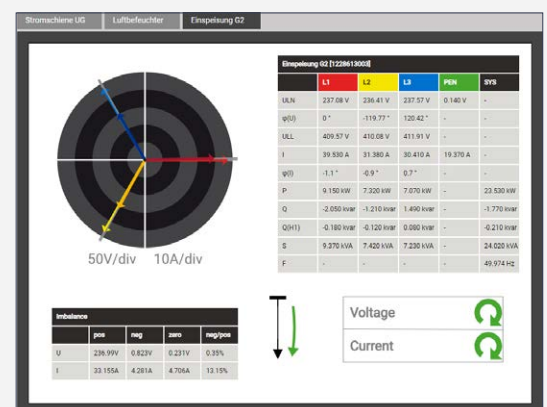
Diagramme vectoriel de contrôle des connexions
