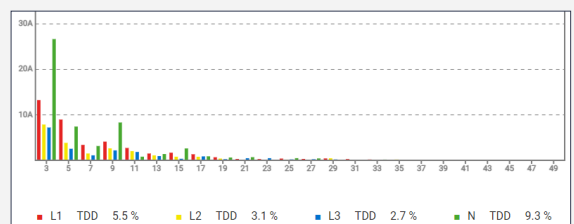
Analyse des harmoniques / interharmoniques pour les 4 courants de chaque module de courant, également disponible sous forme de valeurs moyennes sur 10 minutes
