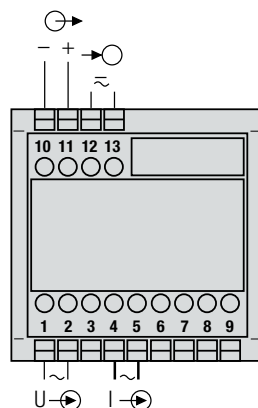
Bild 4. Hilfsenergie-Anschluss auf Niederspannungsseite an Klemmen 12 und 13.
