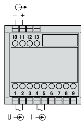
Bild 3. Hilfsenergie intern ab Messeingang, Hilfsenergie-Anschluss entfällt.
