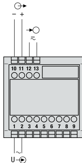
Bild 4. Hilfsenergie-Anschluss auf Niederspannungsseite an Klemmen 12 und 13.
