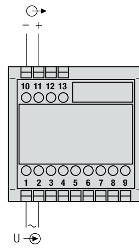
Fig. 3. Alimentation auxiliaire interne, de l'entrée de mesure, sans alimentation auxiliaire.
