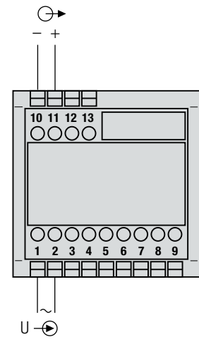
Bild 3. Hilfsenergie intern ab Messeingang, Hilfsenergie-Anschluss entfällt.
