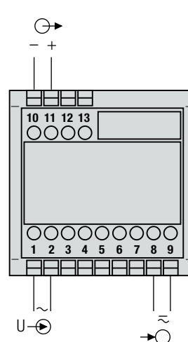
Bild 2. Hilfsenergie-Anschluss an Klemmen 8 und 9.
