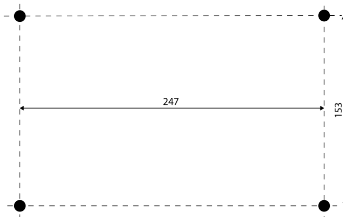
Bohrplan für Feldgehäuse
