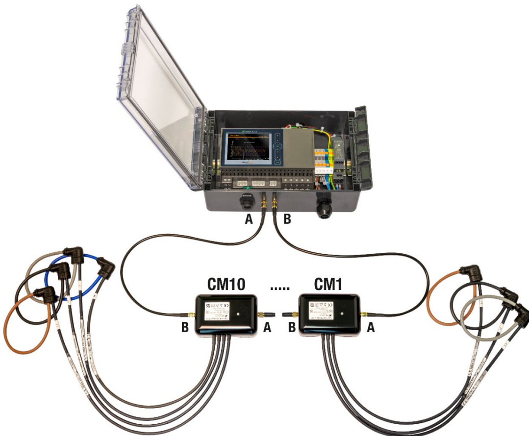
PQ5000CL-3 im Feldgehäuse mit angeschlossenen Current Modulen 3PN und 3P
