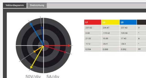
Vektordiagramm zur Anschlusskontrolle
