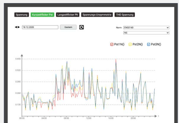
Tagesverlauf des Kurzzeitflickers Pst via Webseite des Gerätes
