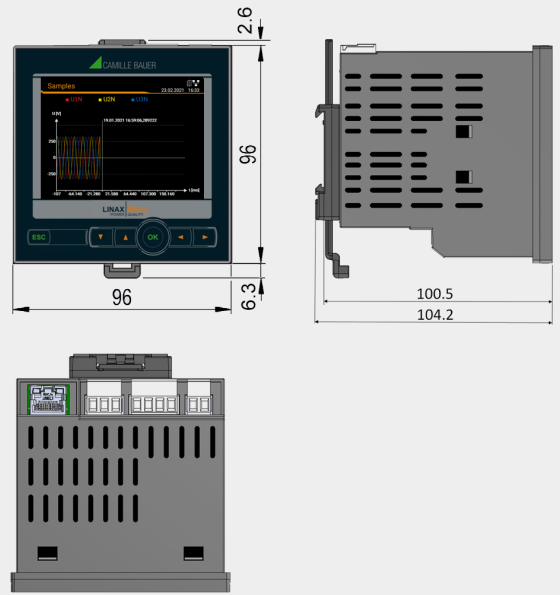
MASSBILD PQ1000-2
