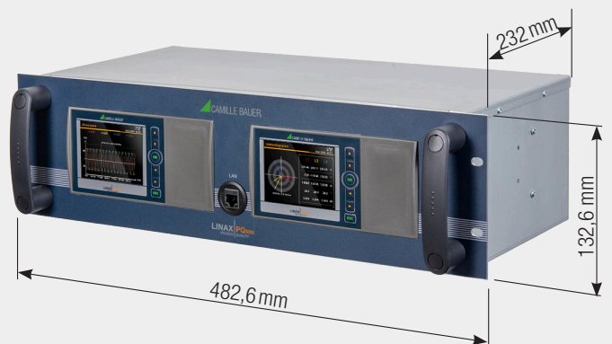
MASSBILD PQ5000-RACK
