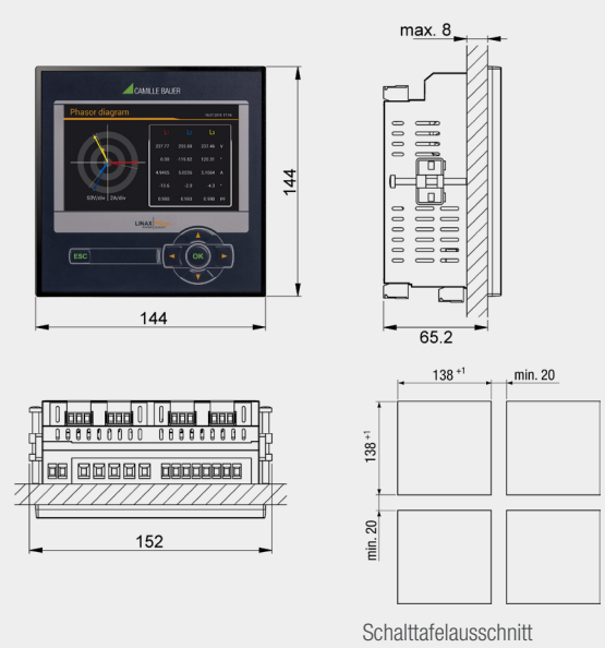
MASSBILD PQ3000
