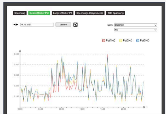
Tagesverlauf des Kurzzeitflickers Pst via Webseite des Gerätes
