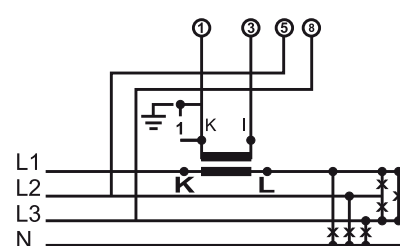
Blindleistungsmessung in einem 3-Phasen, 4-Leiter Netzwerk symetrischer Belastung
