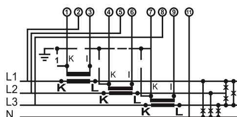
Wirk- und Blindleistungsmessung in einem 3-Phasen, 4-Leiter Netzwerk unsymetrischer Belastung
