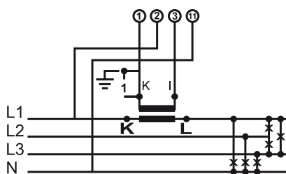
Wirkleistungsmessung in einem 3-Phasen, 4-Leiter Netzwerk symetrischer Belastung
