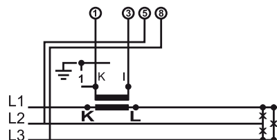
Blindleistungsmessung in einem 3-Phasen, 3-Leiter Netzwerk symetrischer Belastung
