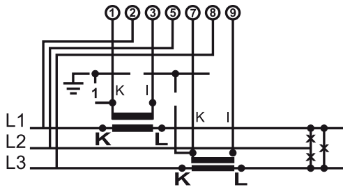
Wirk- und Blindleistungsmessung in einem 3-Phasen, 4-Leiter Netzwerk unsymmetrischer Belastung
