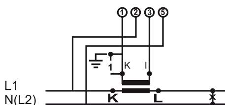
Wirk- und Blindleistungsmessung in einem einphasen Netzwerk
