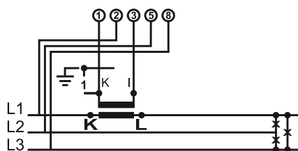
Wirkleistungsmessung in einem 3-Phasen, 3-Leiter Netzwerk symetrischer Belastung
