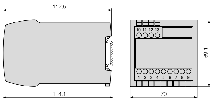
Bild 8. SINEAX U 554 im Gehäuse P13/70 auf Hutschiene (35 × 15 mm oder 35 × 7,5 mm, nach EN 50 022) aufgeschnappt.
