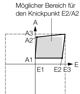
Bild 4. Kennlinie B:
