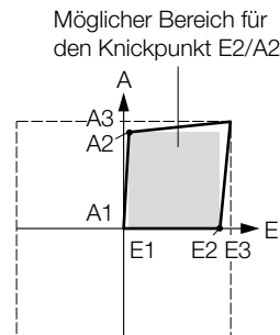
Bild 3. Kennlinie A:
