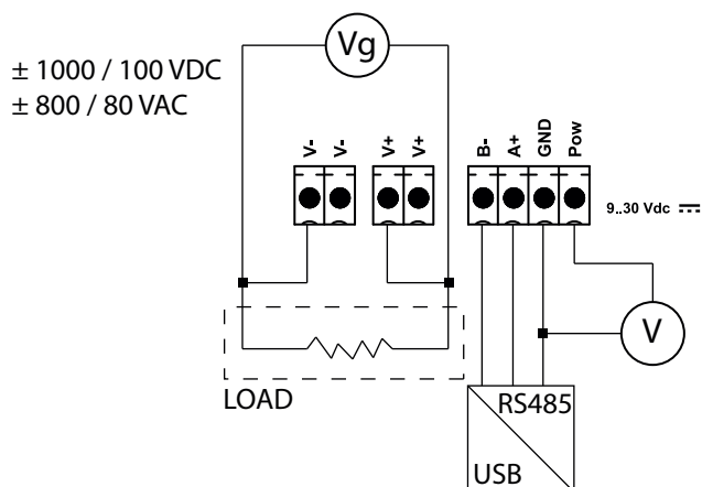
Anschlussschema BT7200 / BT750
