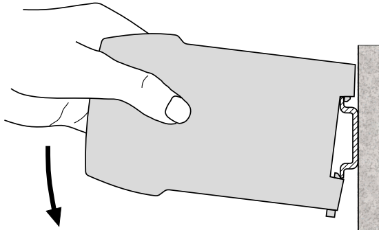
Bild 1. Montage auf Hutschiene 35 x 15 oder 35 x 7,5 mm.
