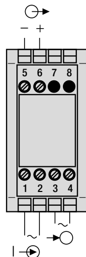
Fig. 2. Alim. auxiliaire CA.
