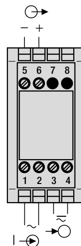
Fig. 5. Alimentation auxiliaire CC, CA en exécution avec bloc d'alim. CC, CA incorporé.
