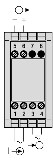
Bild 5. DC-, AC-Hilfsenergie, bei Ausführung mit eingebautem DC-, AC-Netzteil.
