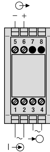
Bild 2. AC-Hilfsenergie.
