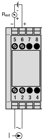
Bild 4. Speisung über Ausgangskreis.
