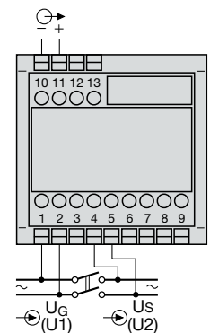
Fig. 3. Alimenté interne par l'entrée de mesure, alimentation auxiliaire pas nécessaire.
