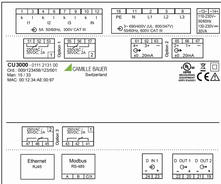
Typenschild eines CU3000 mit
