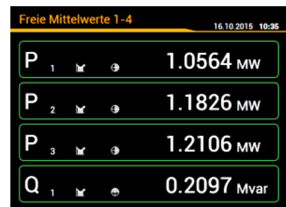
CU5000: Freie Mittelwerte, Trend
