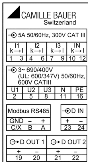
Typenschilder eines CU5000 mit
