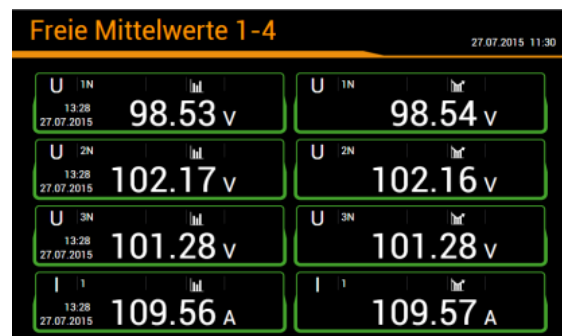
AM3000: Freie Mittelwerte (Letzter Wert und Trend)
